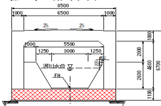
標準断面図
