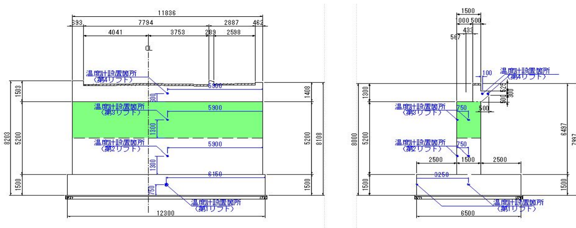
打込みリフト図
