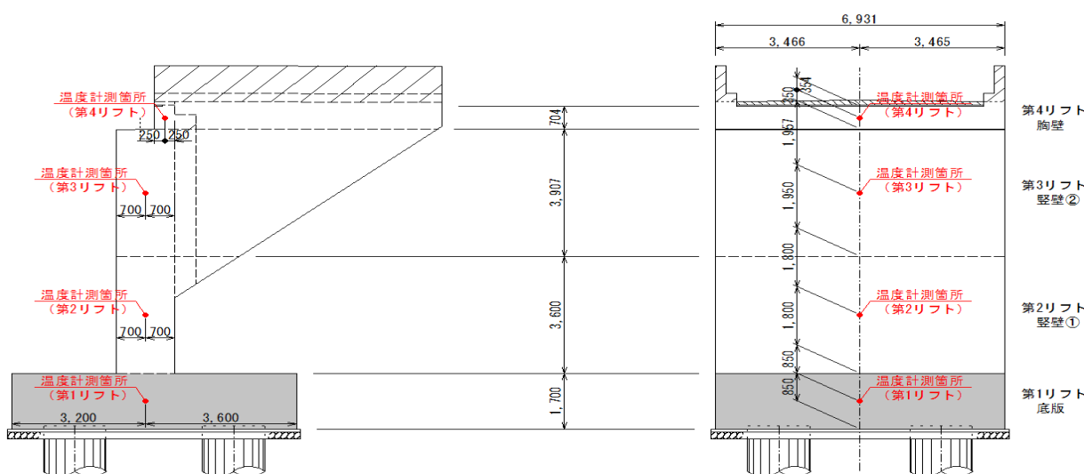
打込みリフト図
