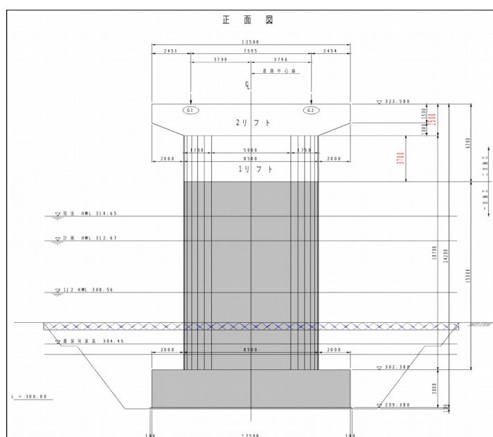
打込みリフト図
