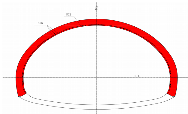
正面図
