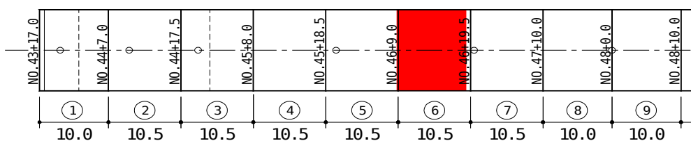
正面図
