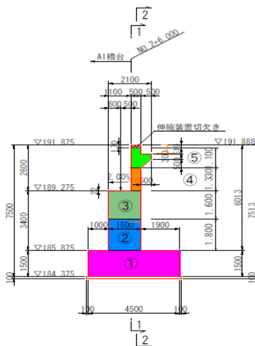
打込みリフト図
