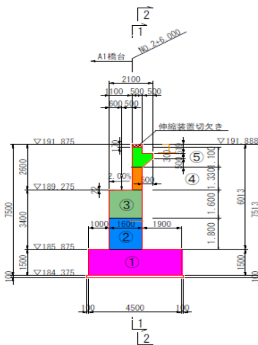
打込みリフト図
