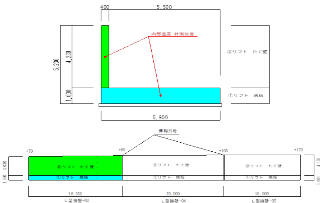
打込みリフト図
