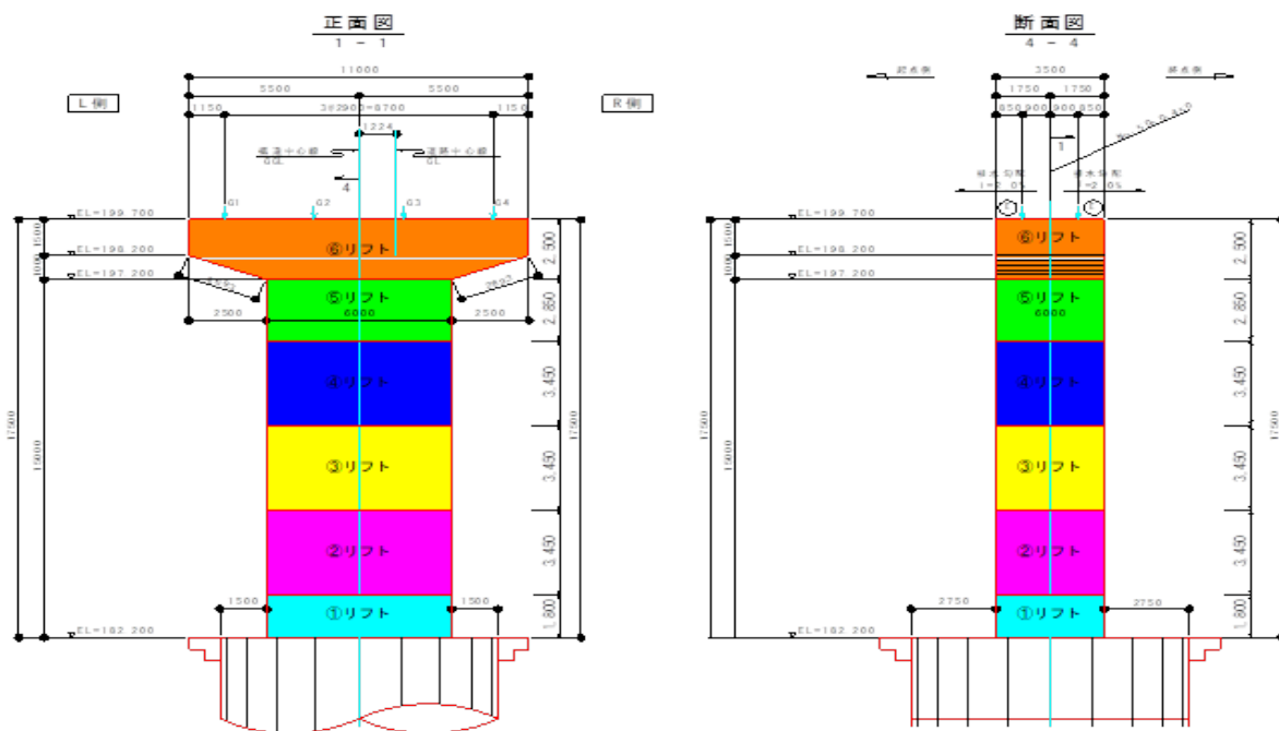
打込みリフト図
